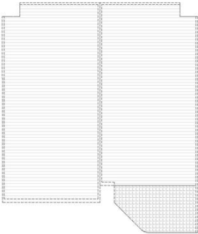
30 Unidades Hab. Double Queen / King : 31.09 m2 (Netos) Hab. Double Queen: 33.10 m2 (Título) 46 Unidades Hab. King: 34.69 m2 (netos) Hab. King: 36.25 m2 (Título) Interior: 28.87 m2 Terraza 5.82 m2
